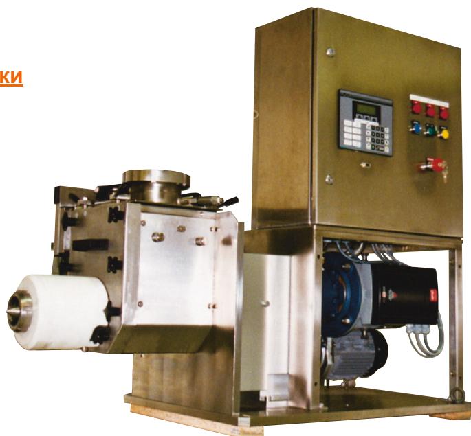
Лабораторный миксер MXE
