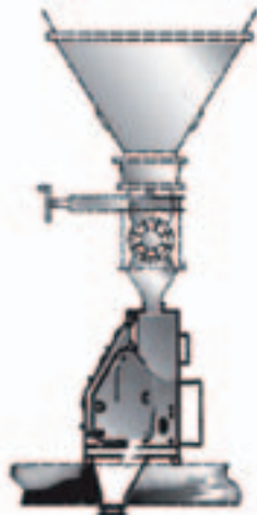
Zellenradschleuse
